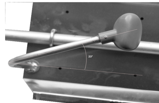
e) Ajuster le tube optique pour obtenir un angle de 23° (les centre de la caméra doit être aligné avec l'axe de la plaque métallique).
