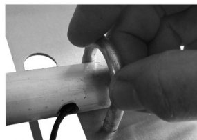
a) Aligner le tube supportant l'antenne avec l'axe de la plaque métallique
